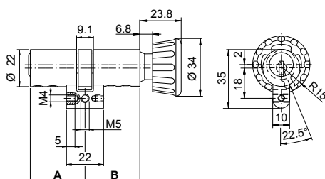
Cylindre à bouton 1519
