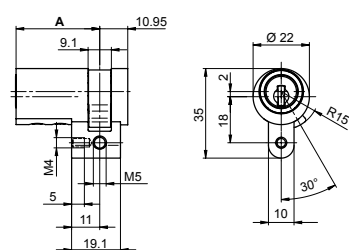
Mezzo cilindro 1514
