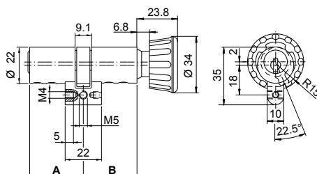
Cilindro con pomello 1519
