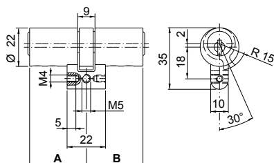
Doppio cilindro 1515
